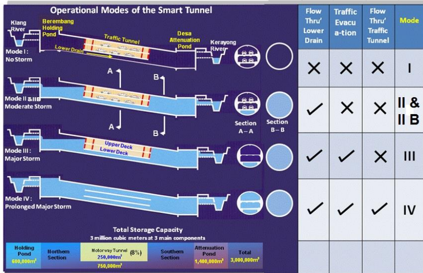
Gambarajah 8.4: Grafik Mod Trafik Terowong SMART
